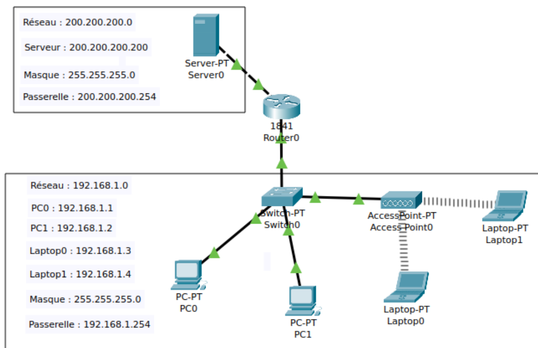
Figure 1. Réseau à base de routeur
